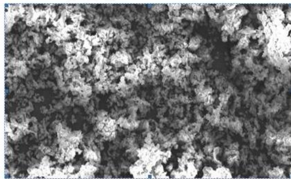
Fig. 4 SEM of Sr S:Eu (0.05)
